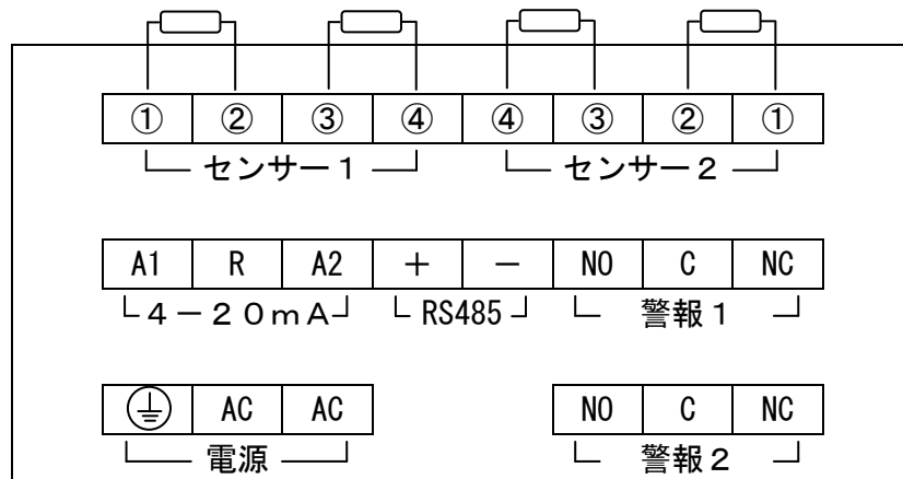
《後面パネル視》
