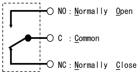
《警報リレー接点説明》
